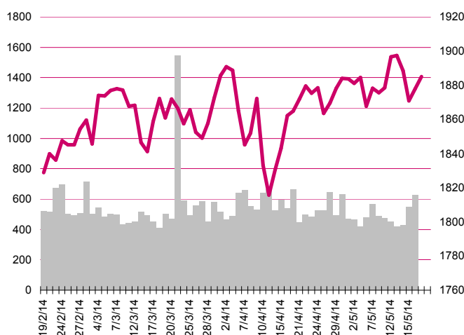
S&P500
