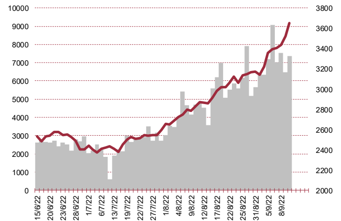
XU100
