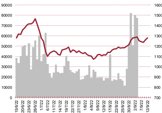
RTSI$
