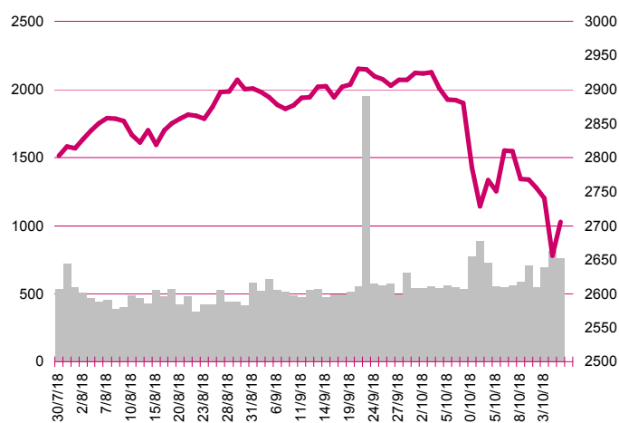
S&P500
